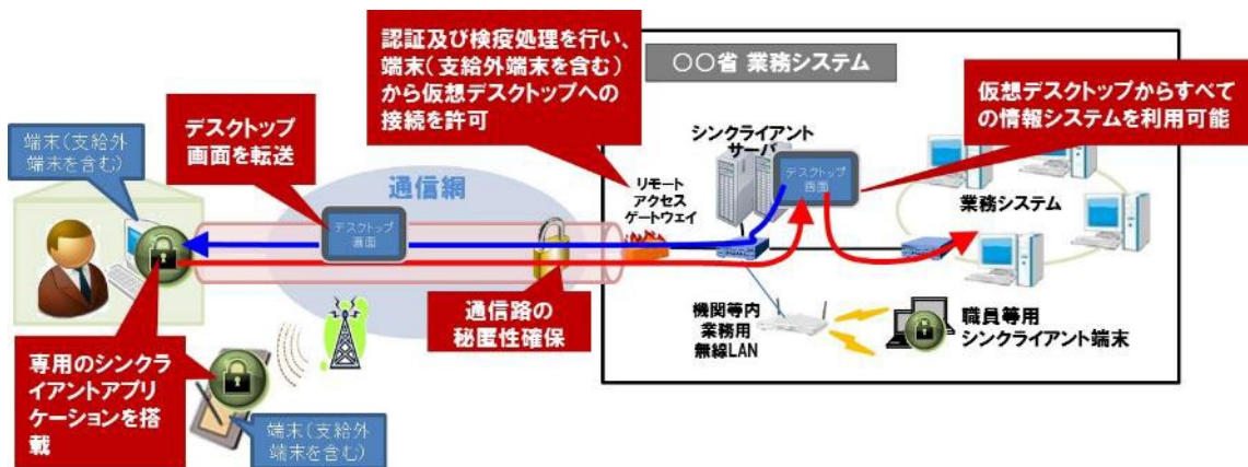
図 6.1.2-1 シンクライアントのシステム構成例
