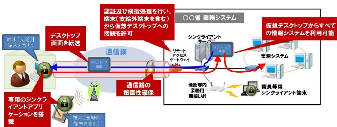
図 7.1.1-1 シンククライアントのシステム構成例
