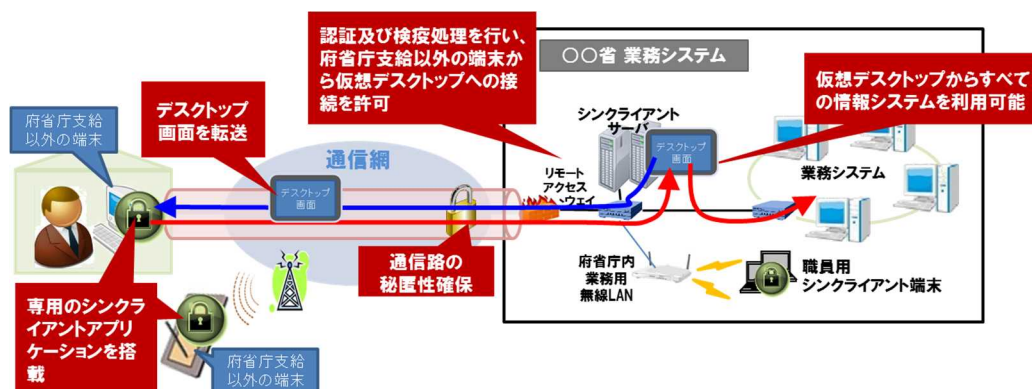
図 8.2.1-1 シンククライアントのシステム構成例
